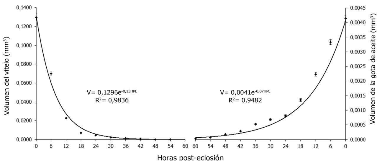
Figura 1. Media ± error estándar de la media en consumo del saco vitelino y gota de aceite de larvas de C. nebulosus / Mean ± standard error mean in yolk sac consumption and oil droplet in larvae of C. nebulosus
